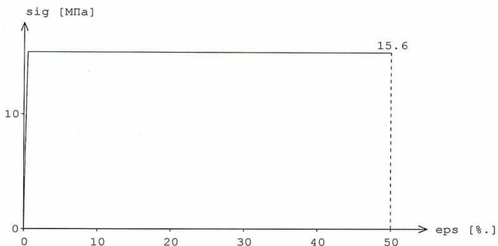
Рис. 8. Диаграмма деформирования s-е бетона при температуре 1000 °С.
