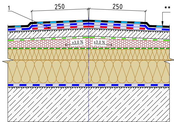
Усиление конька кровли при уклонах поверхности 3 % и более. Задание уклона засыпным материалом по слою теплоизоляции
