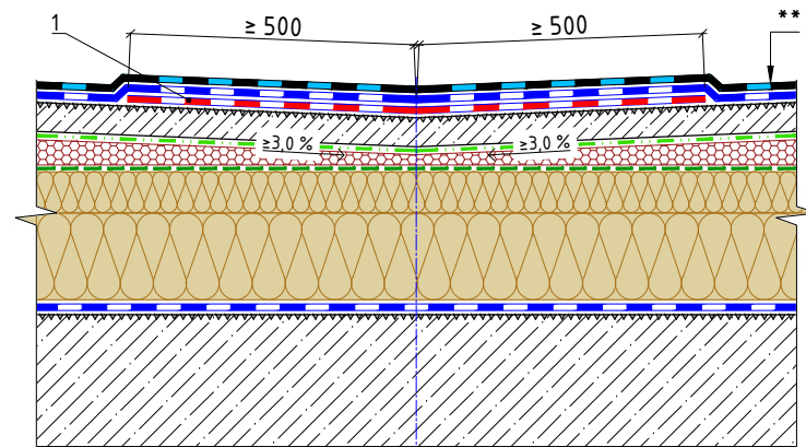
Усиление зоны ендовы кровли при уклонах поверхности 3 % и более.* Задание уклона засыпным материалом по слою теплоизоляции
