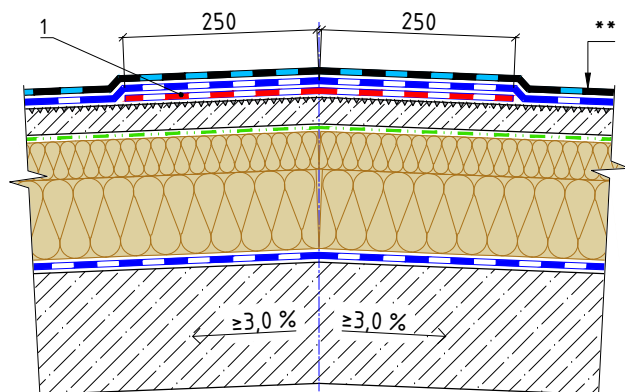
Усиление конька кровли при уклонах поверхности 3 % и более. Задание уклона несущей конструкцией
