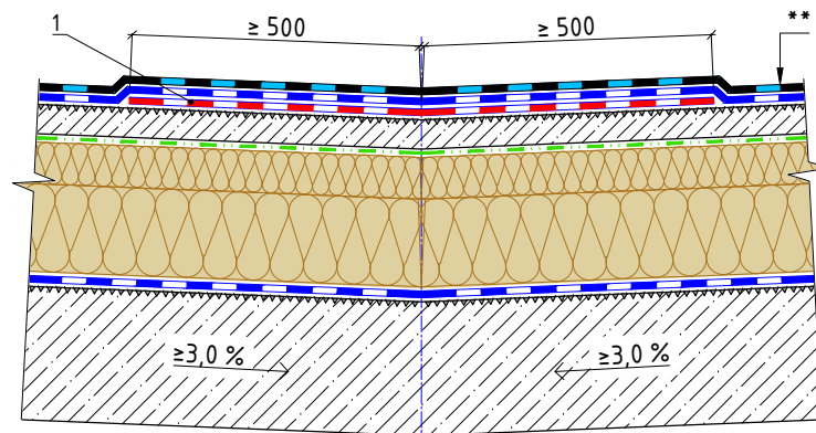
Усиление зоны ендовы кровли при уклонах поверхности 3 % и более.* Задание уклона несущей конструкцией
