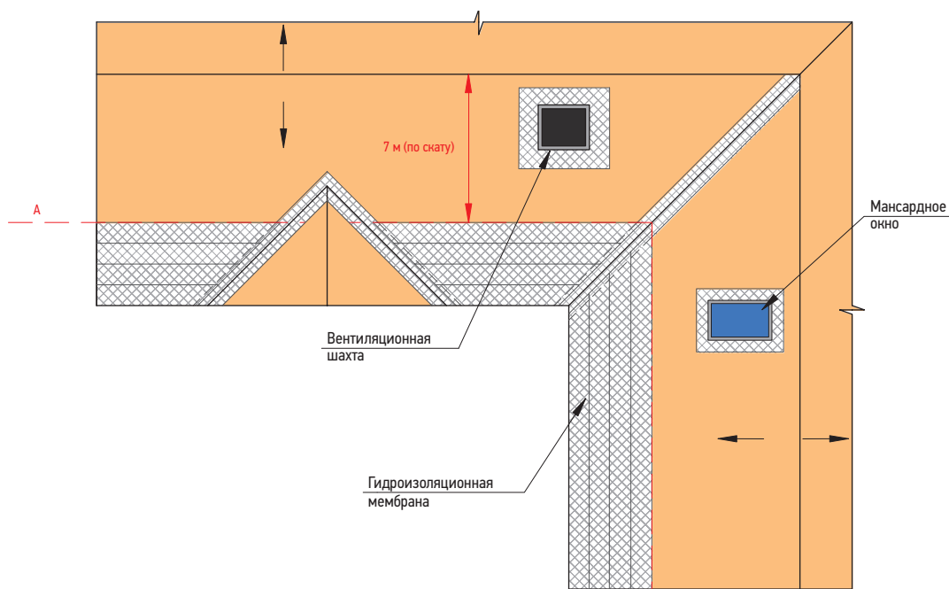
Рис. 2.22. Частичный с дополнительными рядами гидроизоляции по карнизу крыши
